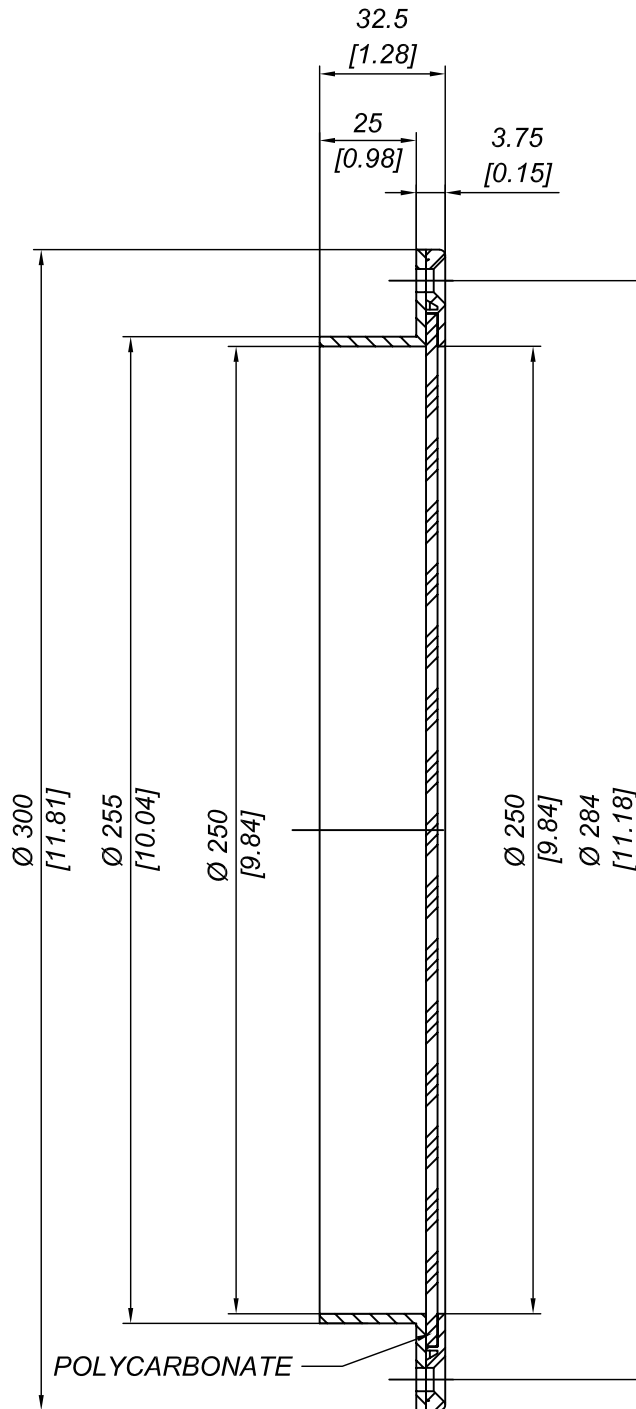
SEZIONE A-A
