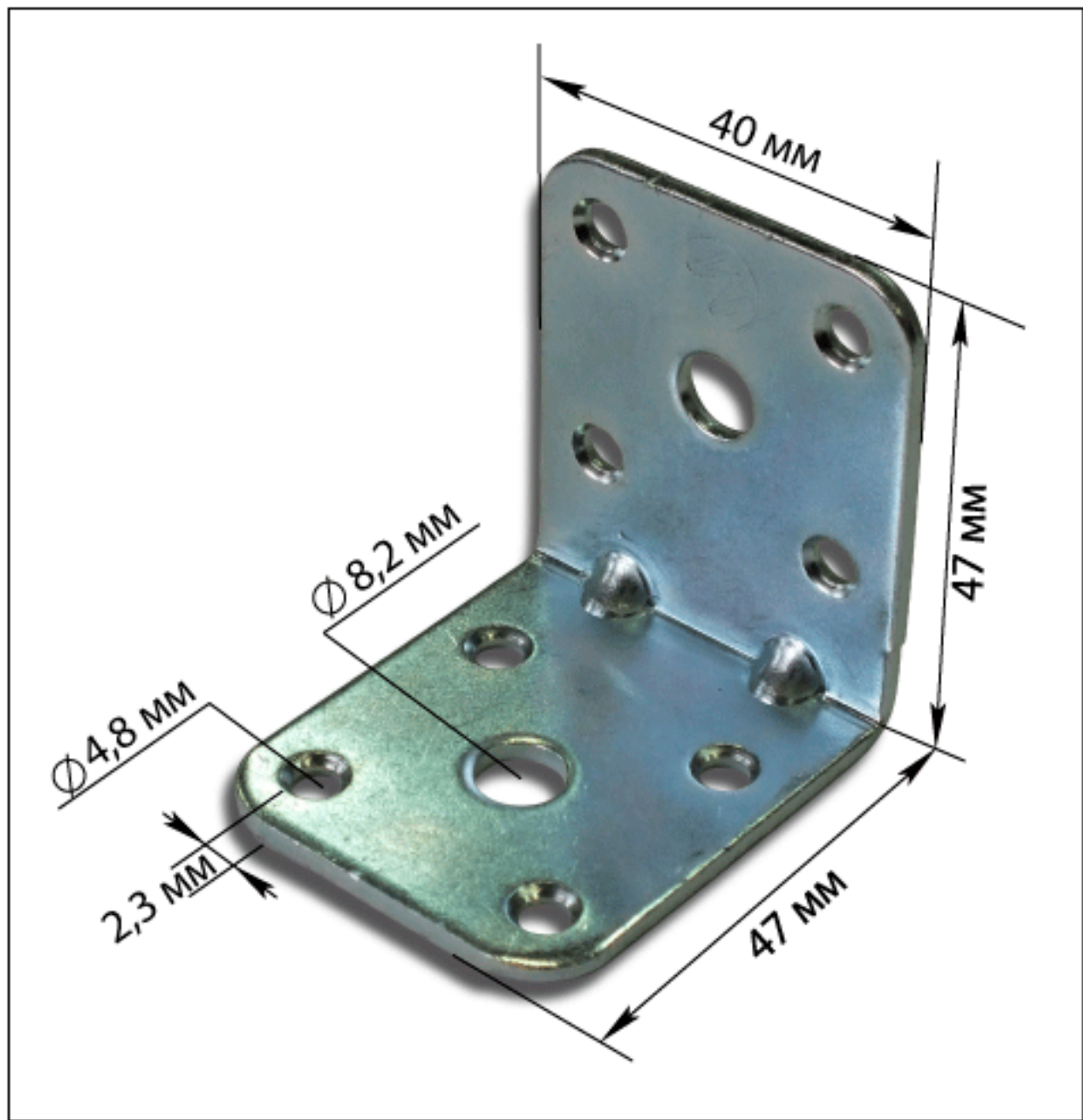
Уголок крепежный 47 x 47 x 40 мм, с 8-ю отв. d 4,8 мм и 2-мя отв. 8,2 мм, оц.ст. 2,3 мм
