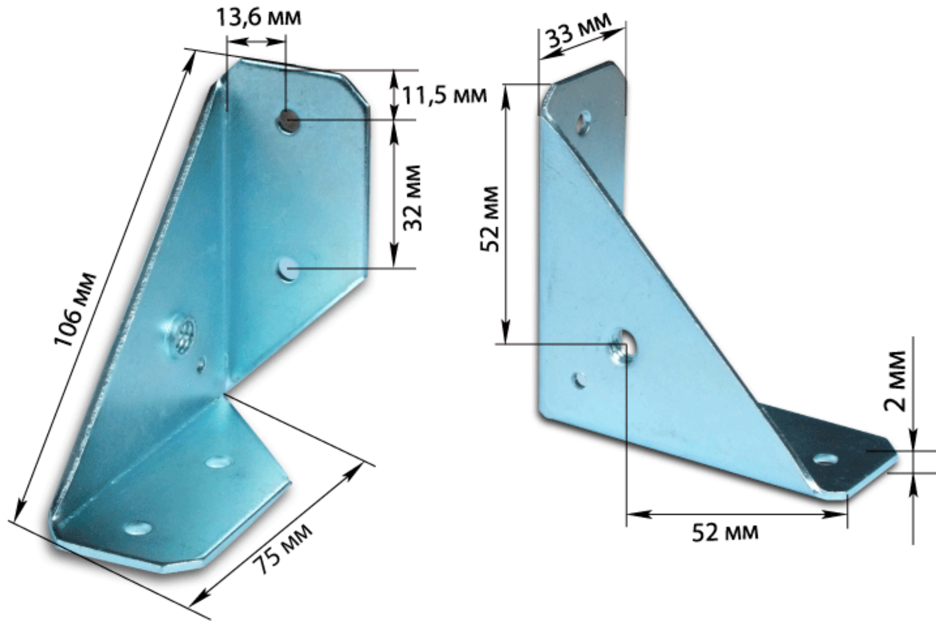
Уголок для стягивания секций 75 x 75 мм
